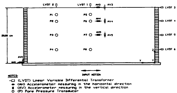
Fig. 2. Centrifuge Model.
